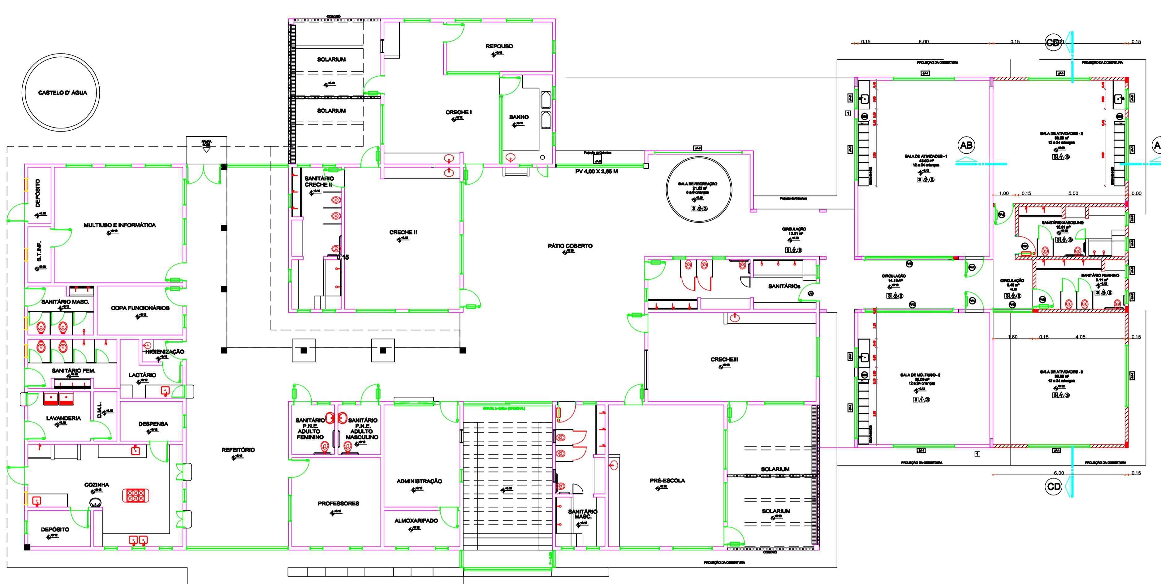
PLANTA BAIXA ESC. 1:100 ÁREA AMPLIAÇÃO: 65,81 M2
